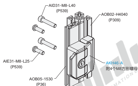
分解图
