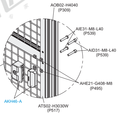
局部放大图
