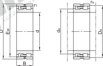
安装图
