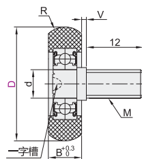
长螺纹型 BKR72
