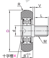
外螺纹型 BKR51 BKR52
