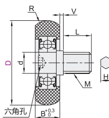
内六角外螺纹型 BKR62
