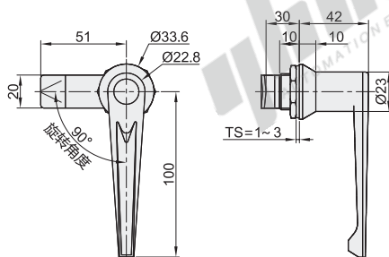
止口高度：30 XAR27
