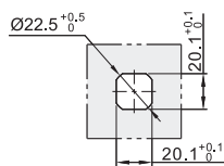
□ 开孔尺寸
