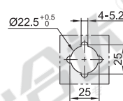
□ 开孔尺寸
