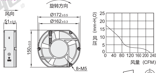
外形尺寸：17251
