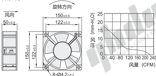
外形尺寸：15050
