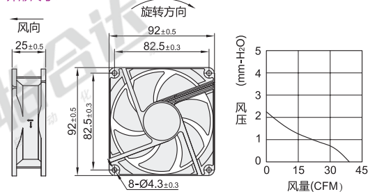
外形尺寸：92
