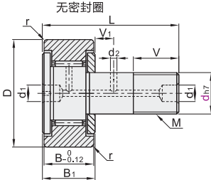
带保持架圆柱型 E-BPC05
