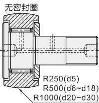
带保持架球面型 E-BPC25
