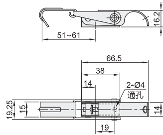
弹簧压缩型 HFQ84
