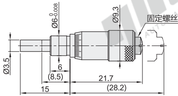
直柄型·平面测量面 EPF02-148-201
