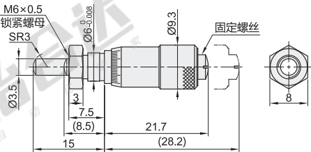
带锁紧螺母·球面测量面 EPF02-148-207
