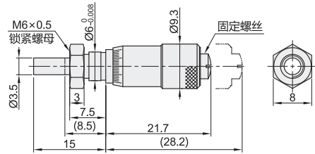
带锁紧螺母·平面测量面 EPF02-148-203
