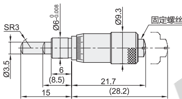
直柄型·球面测量面 EPF02-148-205
