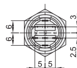
☑ 插脚位置图
