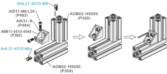
分解图
