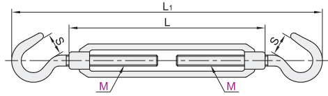
CC型 TCJ92
