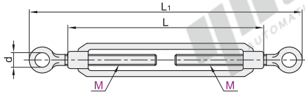
OO型 TCJ91
