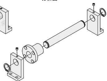
分解图
