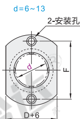
对边法兰型
