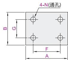
4K(4孔)
