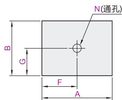
孔加工型 Y-RBB83
