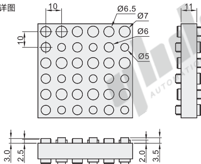
标准型 Y-RBB81
