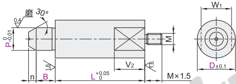
引导型·圆型 YMU41/42/43/44/45/48
