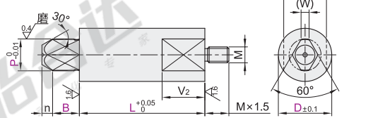
引导型·多棱型 YMU51/52/53/54/55/58
