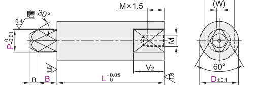
外螺纹型·多棱型 YMU31/32/33/34/35/38
