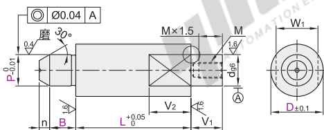
引导型·圆型 YMU41/42/43/44/45/48
