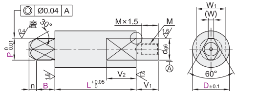
引导型·多棱型 YMU51/52/53/54/55/58
