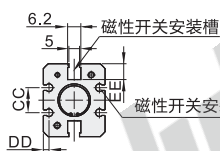
磁性开关安装槽尺寸
