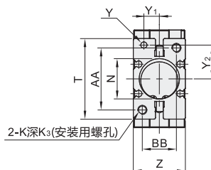
磁性开关安装槽尺寸
