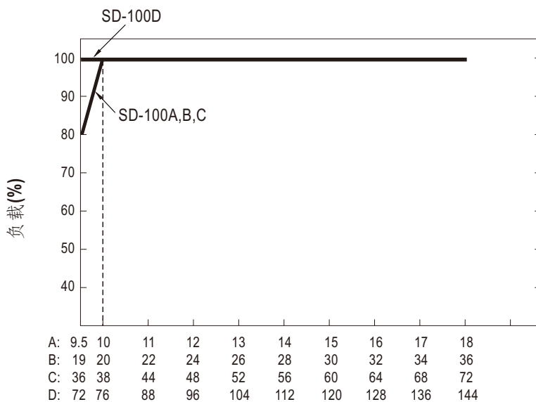
■ 减额输出 VS 输入电压
