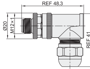
弯式公插头 ZIX13
