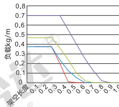
安全塌腰长度与负载关系图FLB
