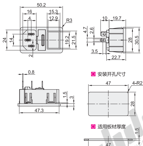
面板安装卡扣型
