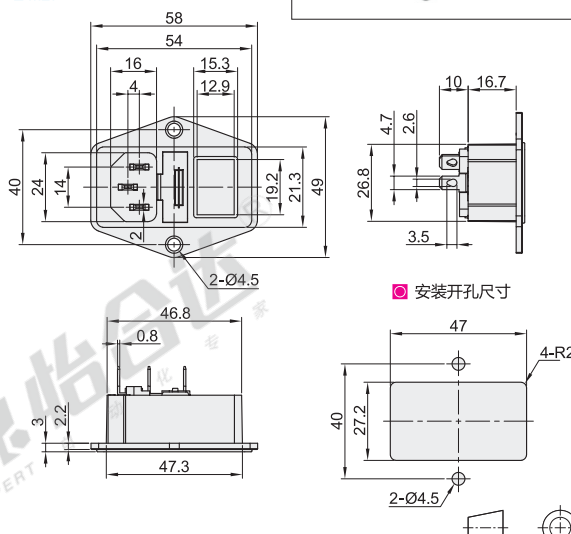
面板安装螺丝固定型
