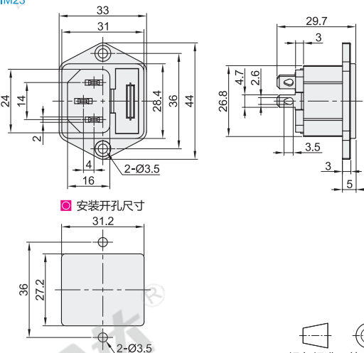
面板安装螺丝固定型
