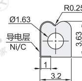
电磁屏蔽型 HGY80
