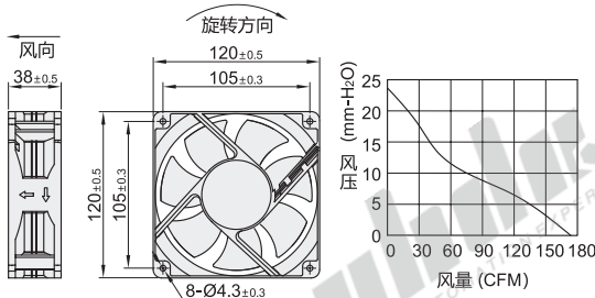
外形尺寸：12038
