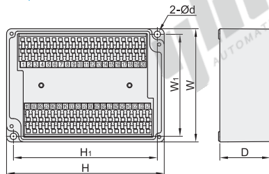
极数: 30P/40P
