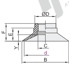
平形 盘径 \phi 10\sim 50
