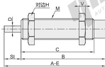
无撞击头 WJG05/06/07
