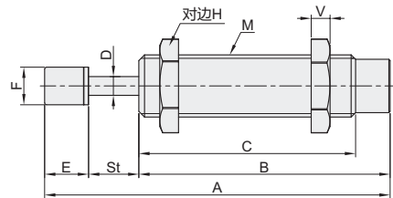
带撞击头 WJG15/16/17
