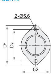
中载型·无垃圾排出孔 QDA10
