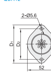
重载型·有垃圾排出孔 QDA12
