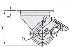
塑胶单刹 CEL41
