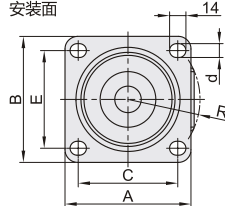
CEL31-D65A/D75A 安装面
