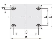
CLB06-D65A/75A 安装面
