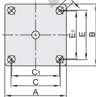
CLB06-D50/65/75 安装面
