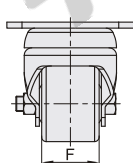
CEL31-D65A/D75A 安装面
