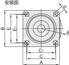
CEL31-D50/65/75 安装面
