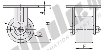
CLB06-D50/65/75 安装面
