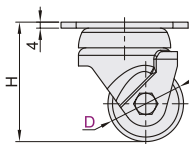
无刹 CEL31
