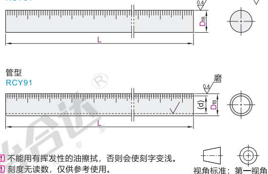
棒型 RCY81
