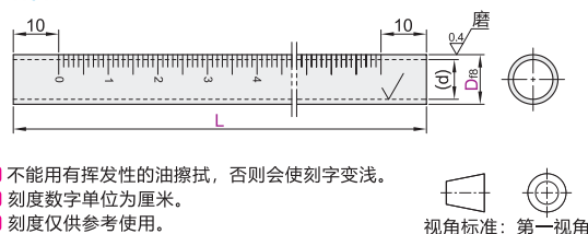
管型 RCY71
