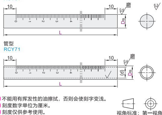
棒型 RCY61
