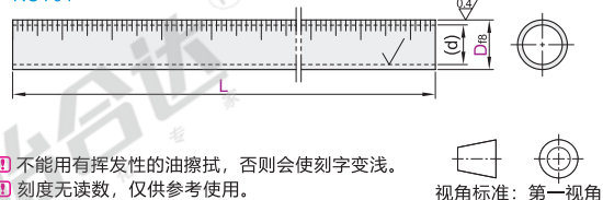
管型 RCY91
