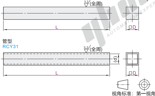
棒型 RCY01
