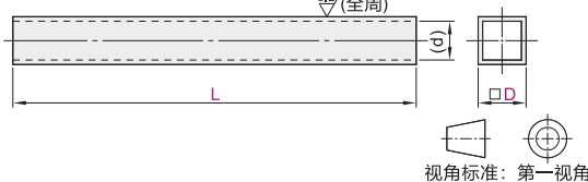
管型 RCY31
