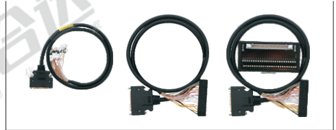
线束+端子台 ZIA16
