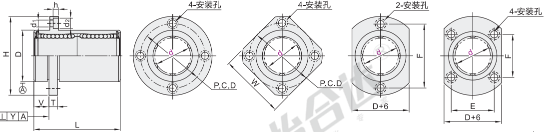
圆法兰型 J-LMK02
