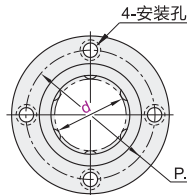
圆法兰型 Y-J-GVD61
