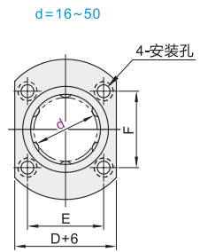
对边法兰型 Y-J-GVD81
