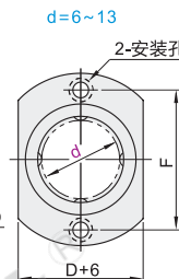
对边法兰型 Y-J-GVD81
