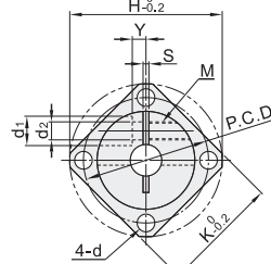
方法兰型 Y-FAE16
