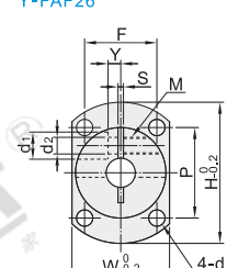
对边法兰型 Y-FAF26
