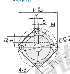
方法兰型 Y-FAF16
