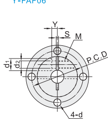
圆法兰型 Y-FAF06
