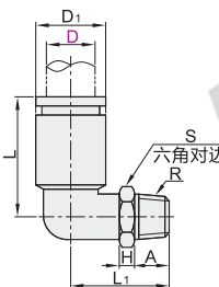
弯接头 XXE01
