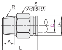
直接头 XXB01
