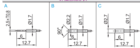
针轴前端形状
