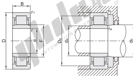
安装图
