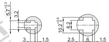
X部放大图 2:1(M3用) Y部放大图 2:1(M6用)
