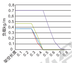
直线架空长度与负载关系图FLG
