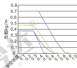
安全塌腰长度与负载关系图FLB
