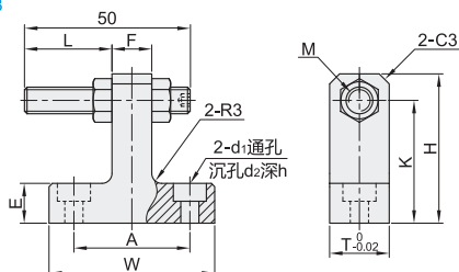
凸型限位块+定位螺栓 ICP53
