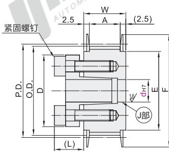
带轮形状
