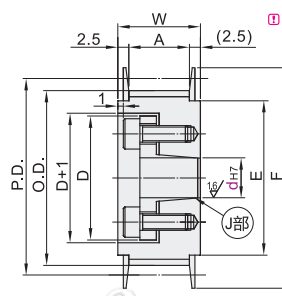
带轮形状
