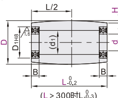
圆弧型 ENL61/71/81/86
