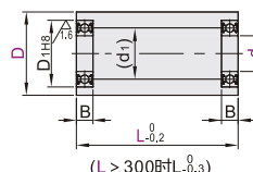
直柱型 ENL01/11/21/26
