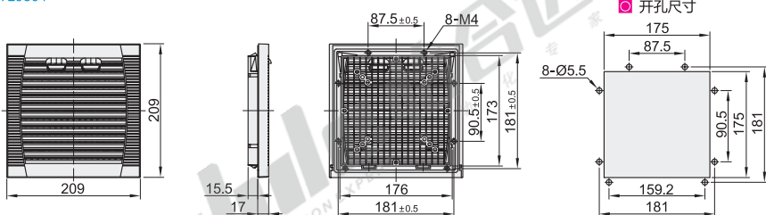
适用风扇尺寸: TL9804
