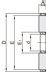
单件 带保持器止推滚针 BKL
