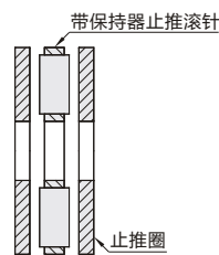
组件 带保持器止推滚针+止推圈 BBL
