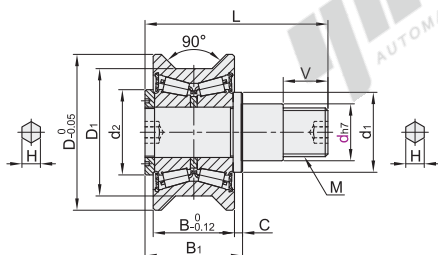
内六角孔型 BPH35
