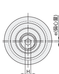
内六角孔偏心型 BPK45
