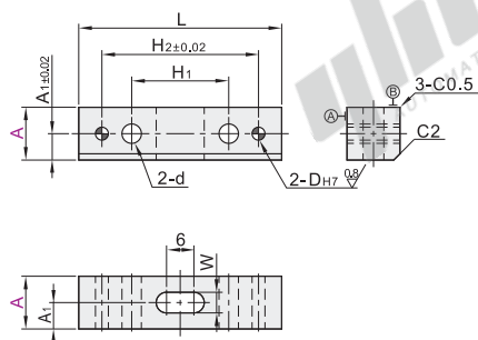
普通型 PDJ01
