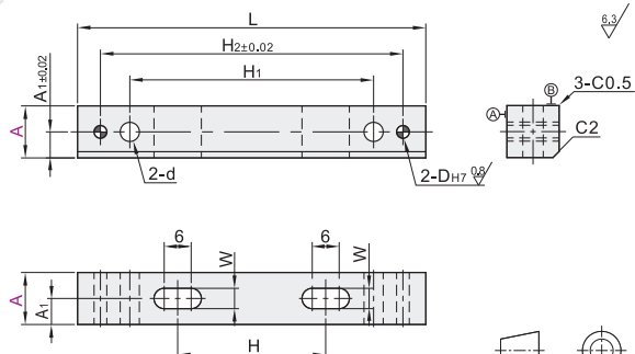
加长型 PDJ06
