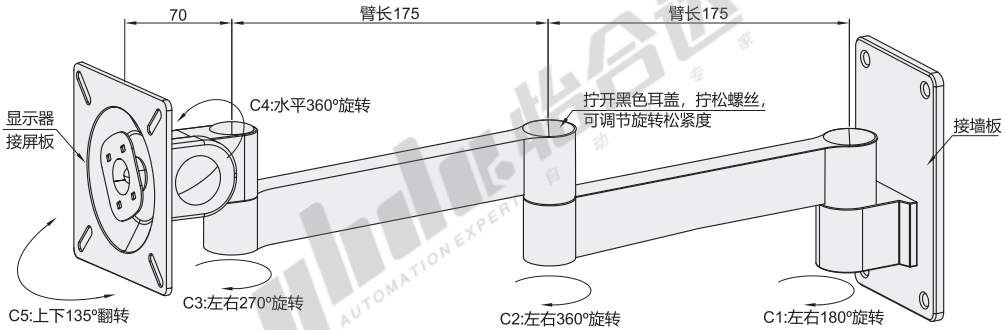
规格: 21 (双臂)
