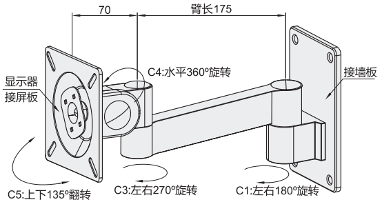
规格: 11 (单臂)
