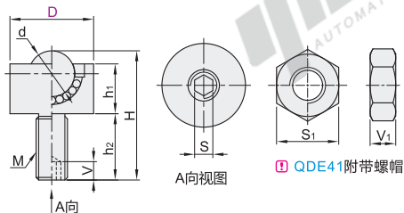
螺帽固定型 QDE41
