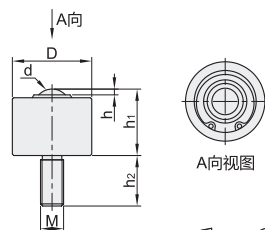
挡圈固定向下使用型 QDE54
