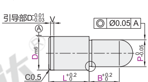
球头型 YPL41/46/51/56
