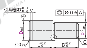
平头型 YPK21/26/31
