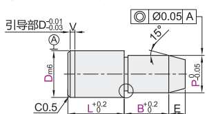
锥角型 YPL01/06/11/16
