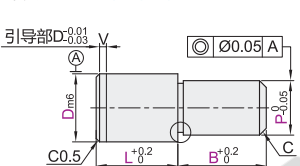
平头型 YPL21/26/31/36
