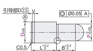
球头型 YPK41/46/51/56
