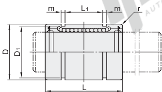
单衬型 Y-GVA01/02/06/07
