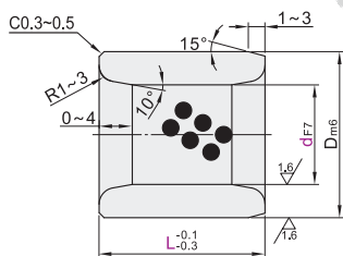
标准型 E-OCK01
