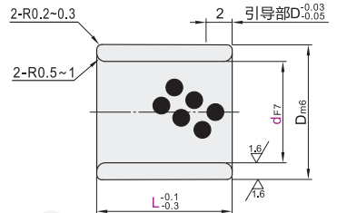
薄壁型 E-OCL01
