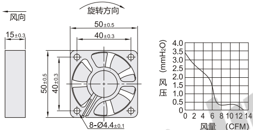
外形尺寸: 5015M2
