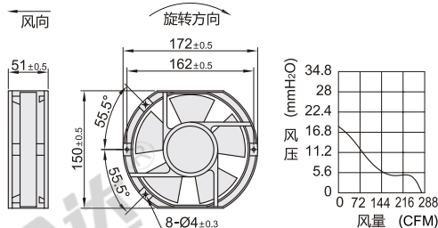
外形尺寸: 17251M2
